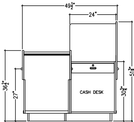
E1 END ELEVATION: SB-142 CHECKOUT L/H SHOWN SCALE: 3/8" = 1'-0"
